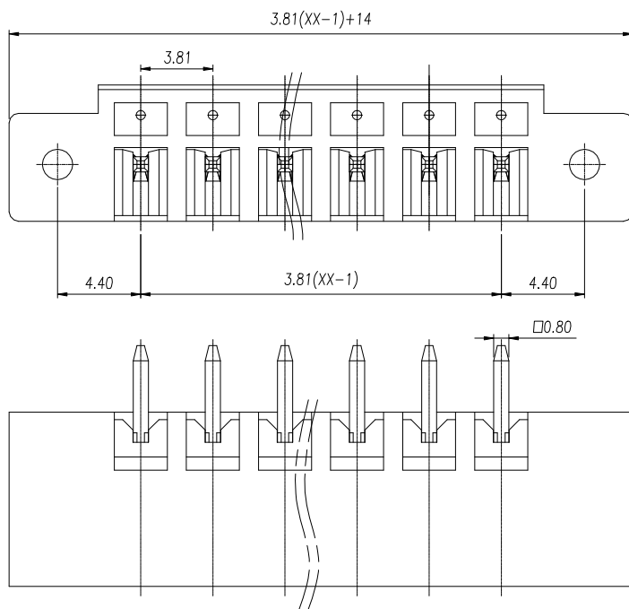
P.C.B. LAYOUT
